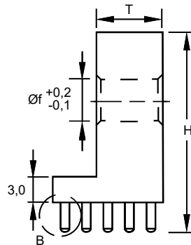
mit Durchgangsloch
