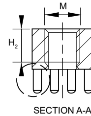
kein Durchgangsgewinde
